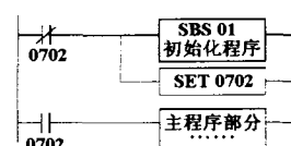
图 3 初始化程序的实现
