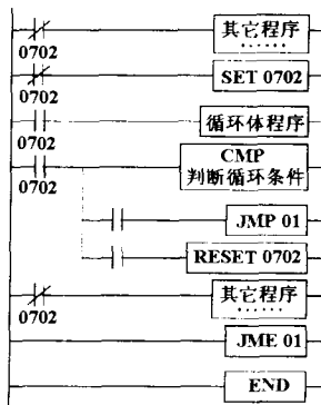
图4 循环的实现
