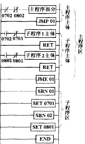
图5 子程序嵌套的实现
